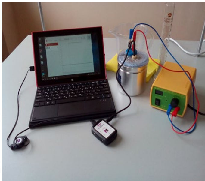
Экспериментальная установка
